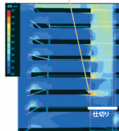
ボイドを利用した温度差換気のシミュレーション例
